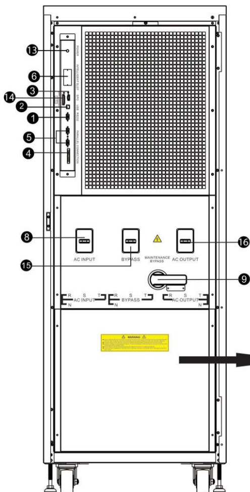
Diagrama 6: Panou deschis față HV 180KT
